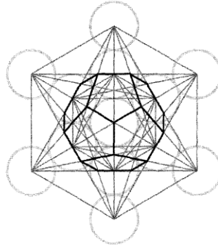
Dodecaedro
