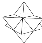
Estrella Tetraédrica
